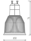
YLD-GU10-7W-G Dorado
